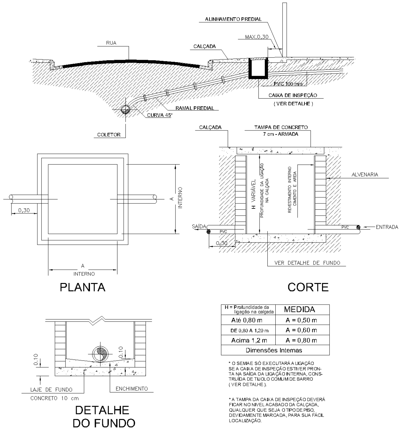
Figura 02: Detalhe da ligação de esgoto
